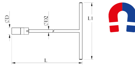
Артикул: 1335 Ключ свечной с шарниром и Т-образной ручкой с магнитной вставкой
