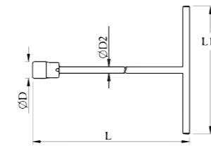
Артикул: 1421 Вороток Т-образный карданный
