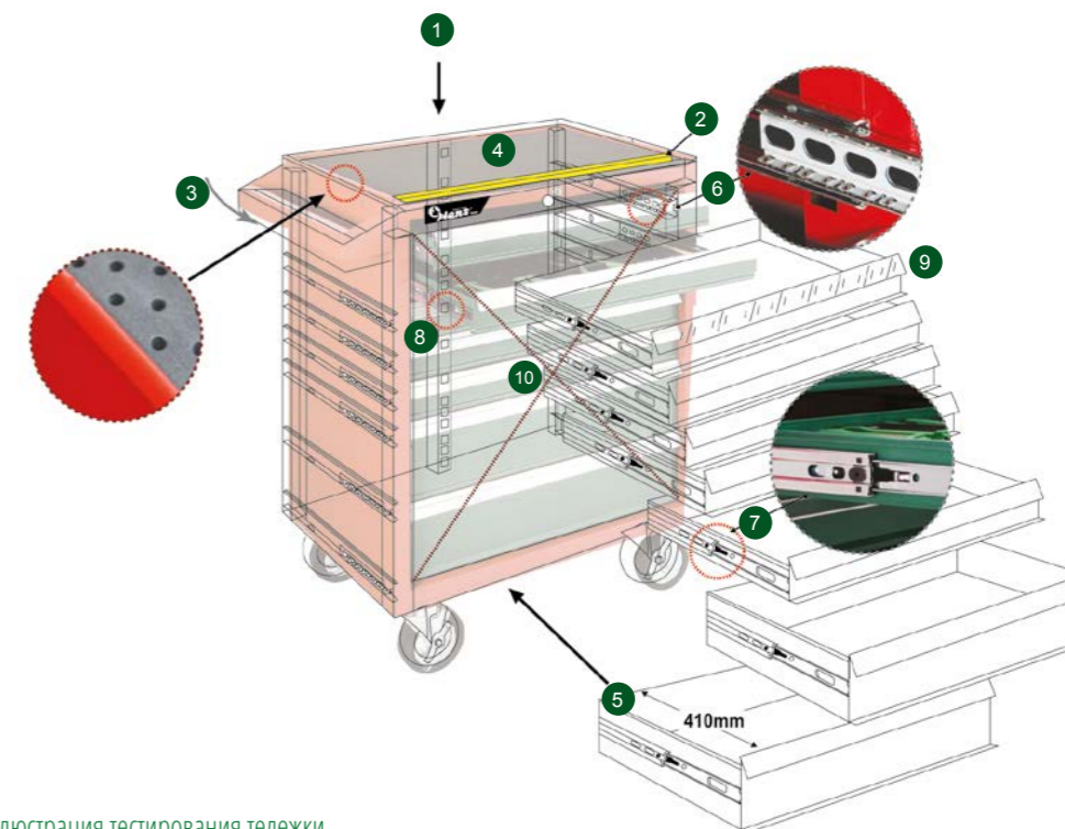
Иллюстрация тестирования тележки HANS 9917HQ под нагрузкой 3650кг.
