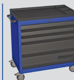
PROFFI 795.5 Размеры (ВхШхГ) 795 x 700 x 490 мм 5 выдвижных ящиков: Средний ящик – 2 шт. Малый ящик – 3 шт.
